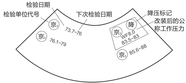
图 4-5 气瓶的检验钢印标记
